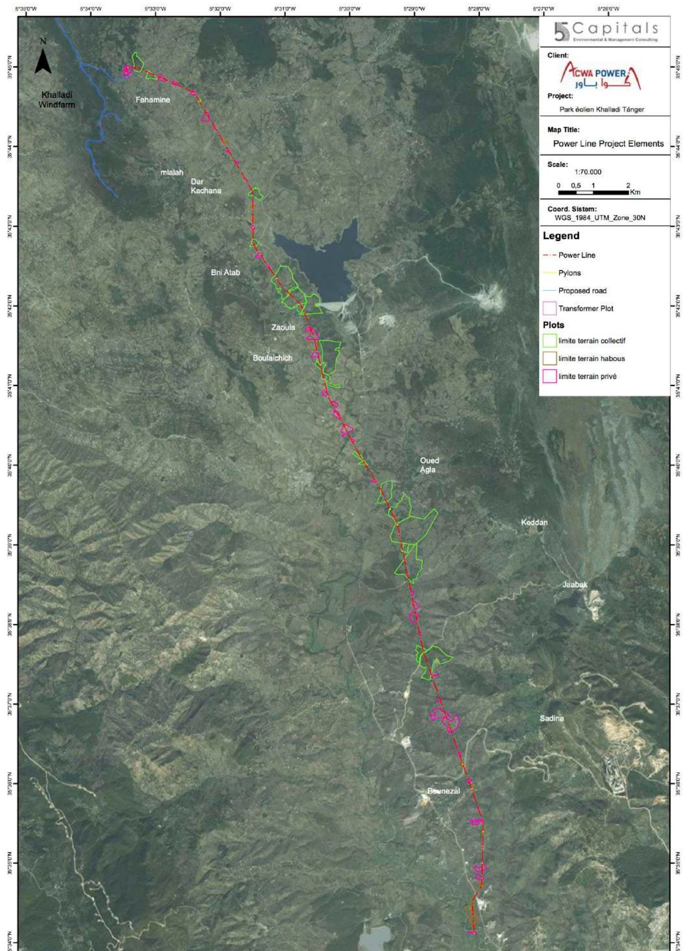
Figure 6: Plan de la ligne Electrique et Utilisations des terres
