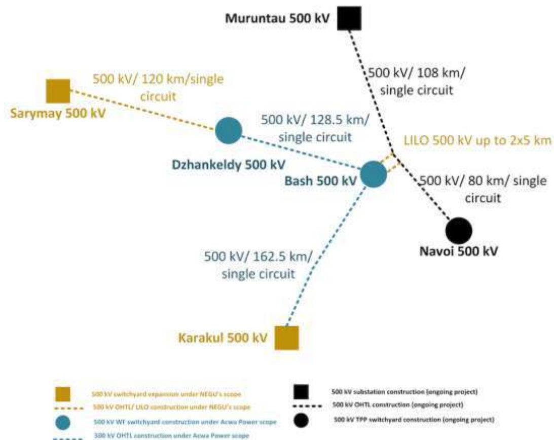
Rasm 2-2 1 GVt quvvatga ega ACWA elektr shamol stansiyalari uchun tarmoqqa ulanish opsiyasi (Jankeldi va Bash)
